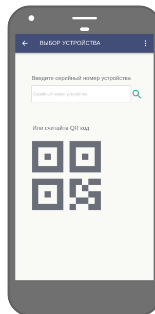
Выбор устройства
