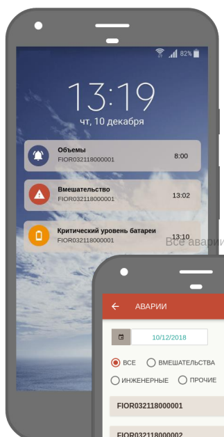
Push уведомления
