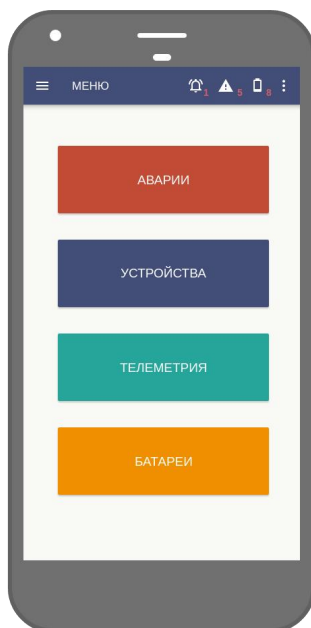
Меню
